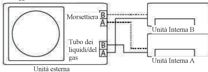
Cablaggio errato
