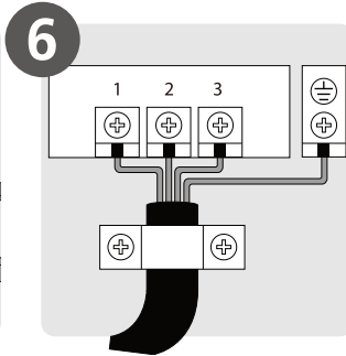
6 Branchement électrique (Page 80)
