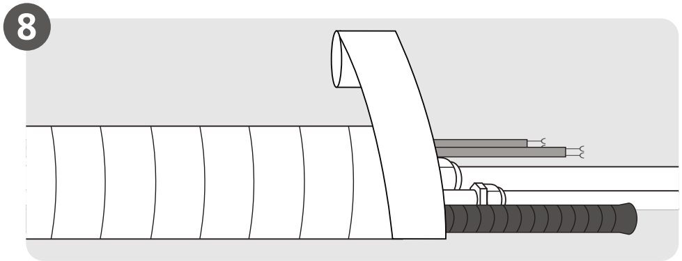
8 Envelopper la tuyauterie et les câbles (Page 83)
