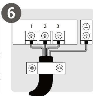
6 Collegare i cavi elettrici (Pagina 139)
