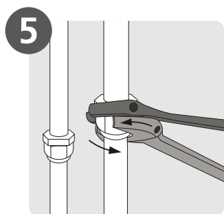
5 Collegare le tubature (Pagina 154)
