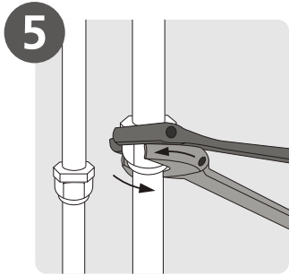
5 Raccorder la tuyauterie (Page 95)
