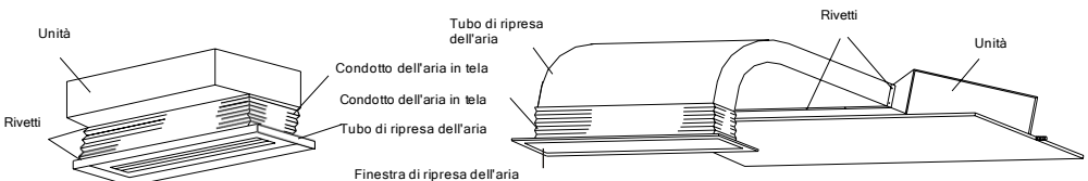
Modalità di installazione per presa d'aria inferiore
