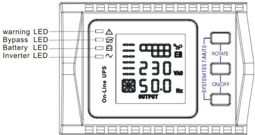
Figura16. Display di controllo UPS
