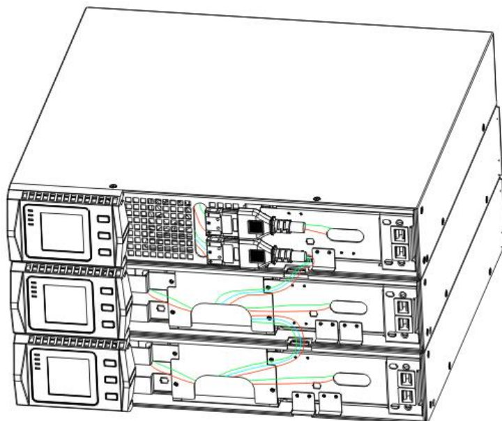
Figure12 Tipica installazione di cabinet batterie (EBP)
