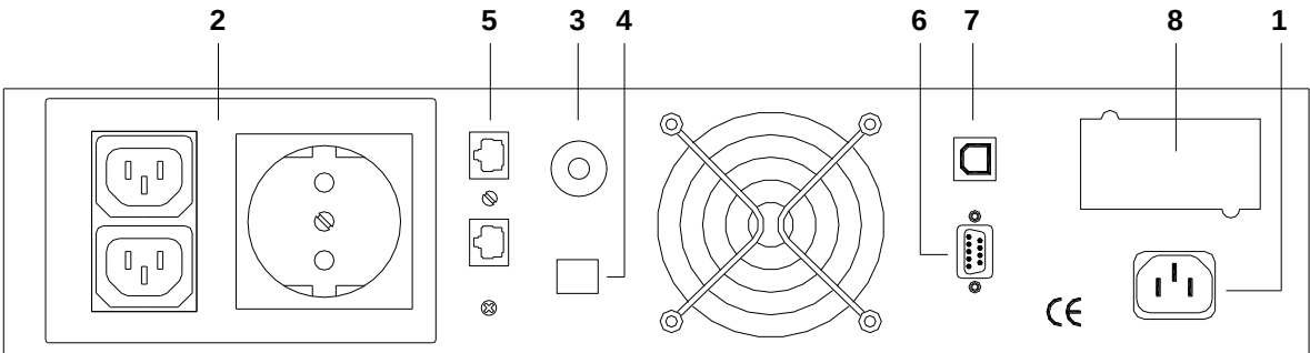
Figura 19 Vista retro dell'UPS
