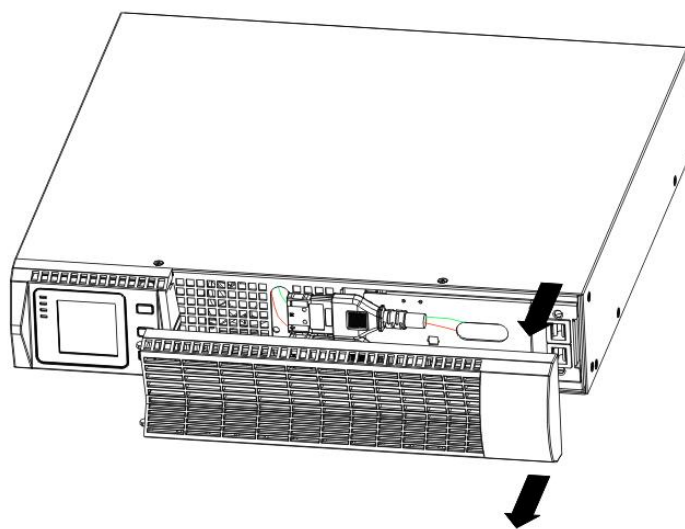
Figura 7 Rimozione frontale UPS
