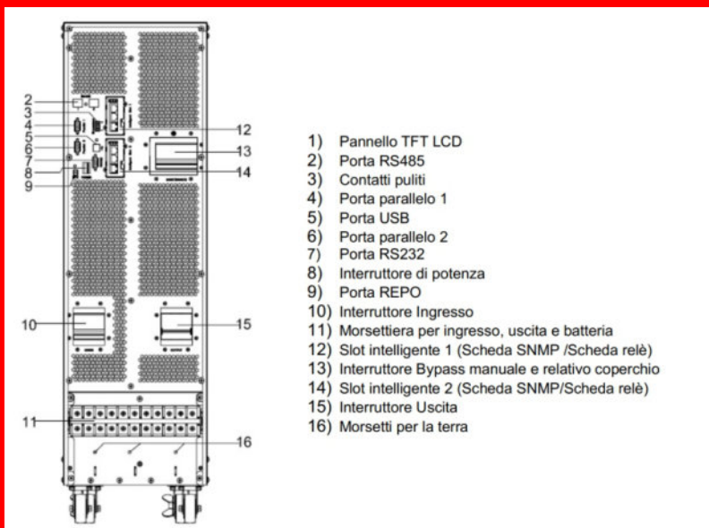
Vista Posteriore 10-20KVA (blocco morsettiere senza coperchio)
